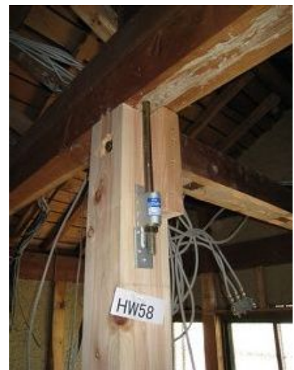
右上柱頭固定金物
