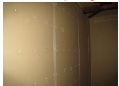
壁・天井下地調整 ジョイントテープ及びビス穴パテ処理
